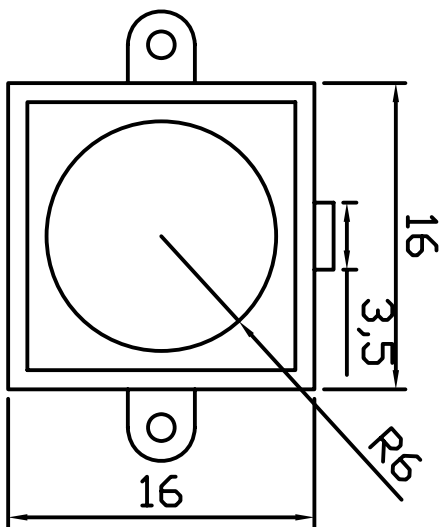
底视图
